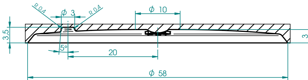
SECTION A-A SCALE 2:1
